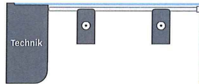
Raucherkabine ST.328-DESIGN für 8 Personen mit 2 Tischmodulen B x T x H in mm: 3280 x 1355 x 2270
