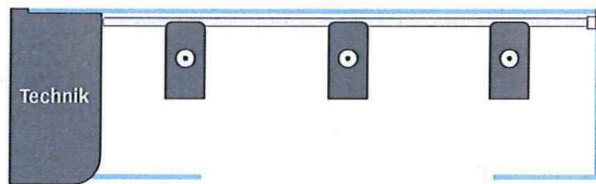
Raucherkabine ST.453-DESIGN für 12 Personen mit 3 Tischmodulen B x T x H in mm: 4530 x 1355 x 227
